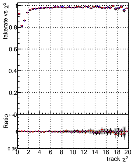
Fake rate vs. DQM mkFit Toriginal DQM mkFit Toriginal DQM mkFit Toriginal DQM mkFit Toriginal DQM mkFit Toriginal DQM mkFit Toriginal DQM mkFit Toriginal DQM mkFit Toriginal DQM mkFit Toriginal DQM mkFit Toriginal DQM mkFit Toriginal DQM mkFit Toriginal DQM mkFit Toriginal DQM mkFit Toriginal DQM mkFit Toriginal DQM mkFit Toriginal DQM mkFit Toriginal DQM mkFit Toriginal DQM mkFit Toriginal DQM mkFit Toriginal DQM mkFit Toriginal DQM mkFit Toriginal DQM mkFit Toriginal DQM mkFit Toriginal DQM mkFit Toriginal DQM mkFit Toriginal DQM mkFit Toriginal DQM mkFit Toriginal DQM mkFit Toriginal DQM mkFit Toriginal DQM mkFit Toriginal DQM mkFit Toriginal DQM mkFit Toriginal DQM mkFit Toriginal DQM mkFit Toriginal DQM mkFit Toriginal DQM mkFit Toriginal DQM mkFit Toriginal DQM mkFit Toriginal DQM mkFit Toriginal DQM mkFit Toriginal DQM mkFit Toriginal DQM mkFit Toriginal DQM mkFit Toriginal DQM mkFit Toriginal DQM mkFit Toriginal DQM mkFit Toriginal DQM mkFit Toriginal DQM mkFit Toriginal DQM mkFit Toriginal DQM mkFit Toriginal DQM mkFit Toriginal DQM mkFit Toriginal DQM mkFit Toriginal DQM mkFit Toriginal DQM mkFit Toriginal DQM mkFit Toriginal DQM mkFit Toriginal DQM mkFit Toriginal DQM mkFit Toriginal DQM mkFit Toriginal DQM mkFit Toriginal DQM mkFit Toriginal DQM mkFit Toriginal DQM mkFit Toriginal DQM mkFit Toriginal DQM mkFit Toriginal DQM mkFit Toriginal DQM mkFit Toriginal DQM mkFit Toriginal DQM mkFit Toriginal DQM mkFit Toriginal DQM mkFit Toriginal DQM mkFit Toriginal DQM mkFit Toriginal DQM mkFit Toriginal DQM mkFit Toriginal DQM mkFit Toriginal DQM mkFit Toriginal DQM mkFit Toriginal DQM mkFit Toriginal DQM
