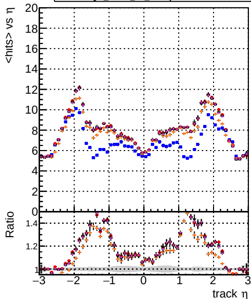
Legend: DQM mkFit TT original, DQM mkFit TT JanUpdate-noErr, DQM mkFit TT JanUpdate-statErr, DQM mkFit TT JanUpdate-systErr, DQM mkFit TT JanUpdate-bothErr mean hit
