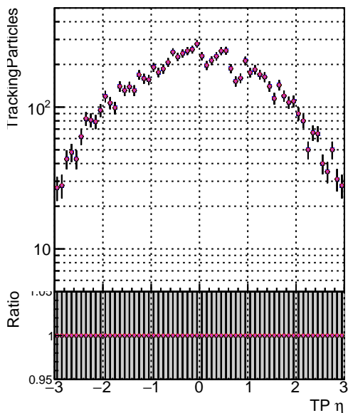
Legend: Blue square: DQM mkFit TToriginal Red circle: DQM mkFit TT JanUpdate-noErr Black triangle: DQM mkFit TT JanUpdate-statErr Orange diamond: DQM mkFit TT JanUpdate-systErr Purple star: DQM mkFit TT JanUpdate-bothErr
