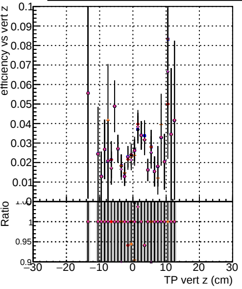
Efficiency vs vertpos DOM mkFit TT Original DOM mkFit TT JanUpdate-noErr DOM mkFit TT JanUpdate-statErr DOM mkFit TT JanUpdate-systErr DOM mkFit TT JanUpdate-bothErr
