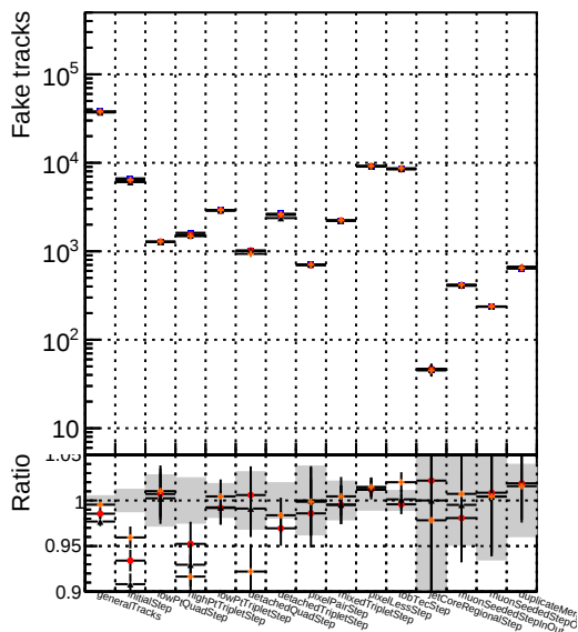
Number —▲— DQM_mkFit_TT_JanUpdate-statErr —◆— DQM_mkFit_TT_JanUpdate-systErr
