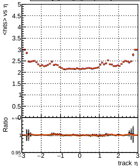
DQM_mkFit_TT_Original DQM_mkFit_TT_JanUpdate-noErr DQM_mkFit_TT_JanUpdate-statErr DQM_mkFit_TT_JanUpdate-systErr
