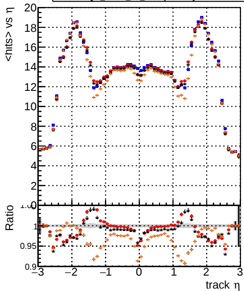
DQM_mkFit_TT_original DQM_mkFit_TT_JanUpdate-noErr DQM_mkFit_TT_JanUpdate-statErr DQM_mkFit_TT_JanUpdate-systErr mean hit
