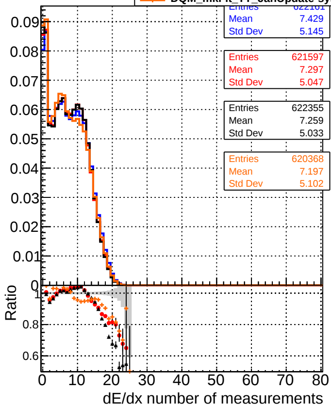
—●— DQM_mkFit_TToriginal —●— DQM_mkFit_TT_JanUpdate-noErr —●— DQM_mkFit_TT_JanUpdate-statErr —●— DQM_mkFit_TT_JanUpdate-systErr
