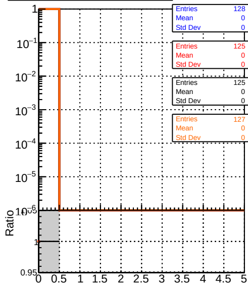
mean hit DQM_mkFit_TT_Original DQM_mkFit_TT_JanUpdate-noErr DQM_mkFit_TT_JanUpdate-statErr DQM_mkFit_TT_JanUpdate-systErr
