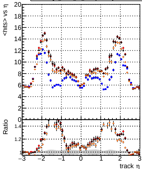
mean hit DQM_mkFit_TT_Original DQM_mkFit_TT_JanUpdate-noErr DQM_mkFit_TT_JanUpdate-statErr DQM_mkFit_TT_JanUpdate-systErr
