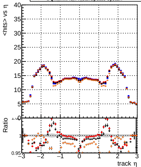
mean hit DQM_mkFit_TT_Original DQM_mkFit_TT_JanUpdate-noErr DQM_mkFit_TT_JanUpdate-statErr DQM_mkFit_TT_JanUpdate-systErr
