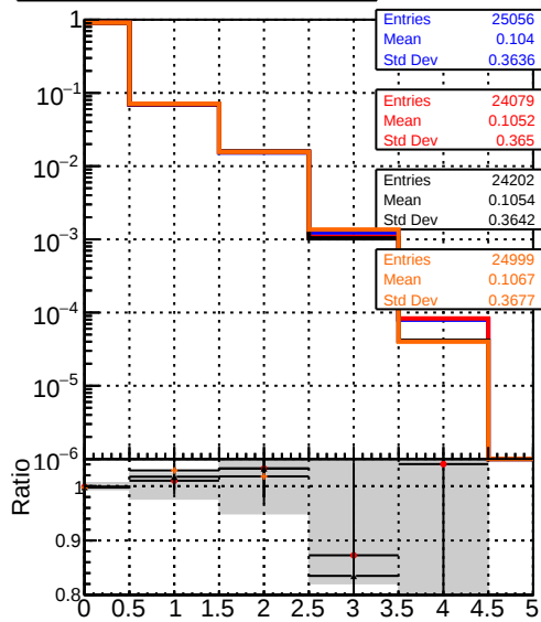
DQM_mkFit_TToriginal DQM_mkFit_TT_JanUpdate-noErr DQM_mkFit_TT_JanUpdate-statErr DQM_mkFit_TT_JanUpdate-systErr mean hit
