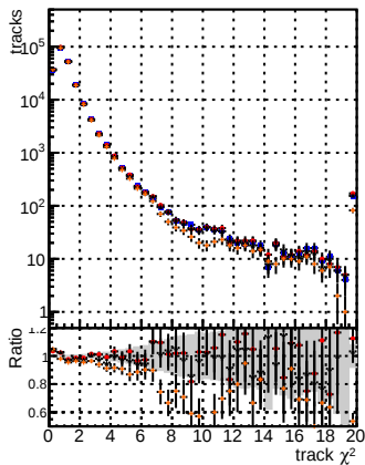
N of reco track vs. BGM HKREIT JanUdate noErr BGM HKREIT JanUdate noErr BGM HKREIT JanUdate svsterr
