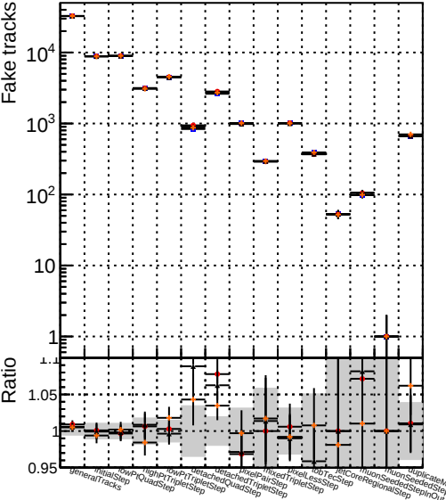
Number Legend 1 —▲— DQM_mkFit_TT_JanUpdate-statErr 2 —♦— DQM_mkFit_TT_JanUpdate-systErr
