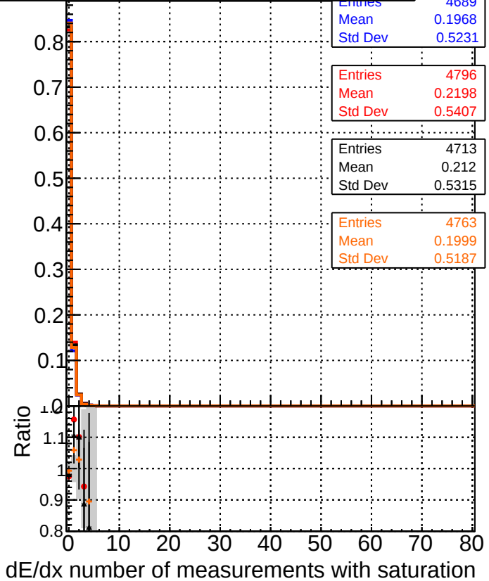
—●— DQM_mkFit_TToriginal —●— DQM_mkFit_TT_JanUpdate-noErr —●— DQM_mkFit_TT_JanUpdate-statErr —●— DQM_mkFit_TT_JanUpdate-systErr
