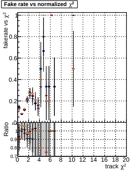
Fake rate vs. BQM mkFit TToOriginal TToUpdateSystem
