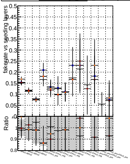
Fake rate vs. BQM mkFit TToOriginal TToUpdateSystem
