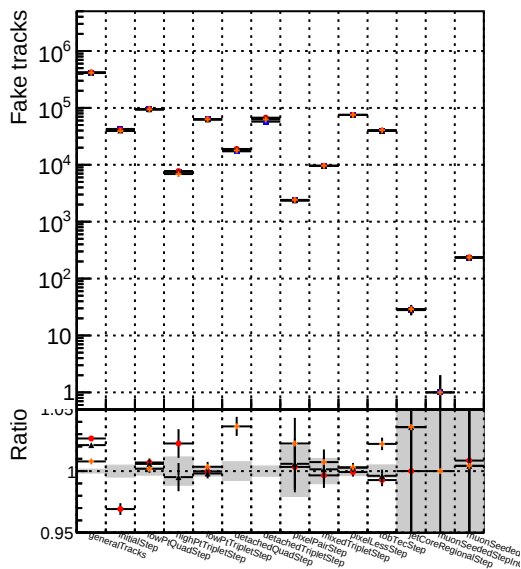
Number Legend —▲— DQM_mkFit_TT_JanUpdate-statErr —+— DQM_mkFit_TT_JanUpdate-systErr
