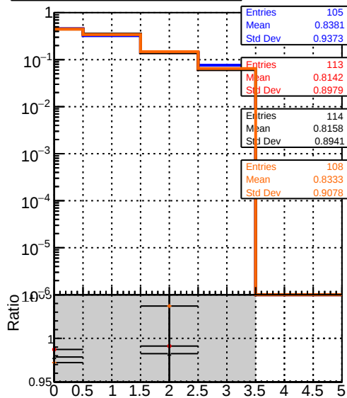
— DQM_mkFit_TToriginal — DQM_mkFit_TT_JanUpdate-noErr — DQM_mkFit_TT_JanUpdate-statErr — DQM_mkFit_TT_JanUpdate-systErr
