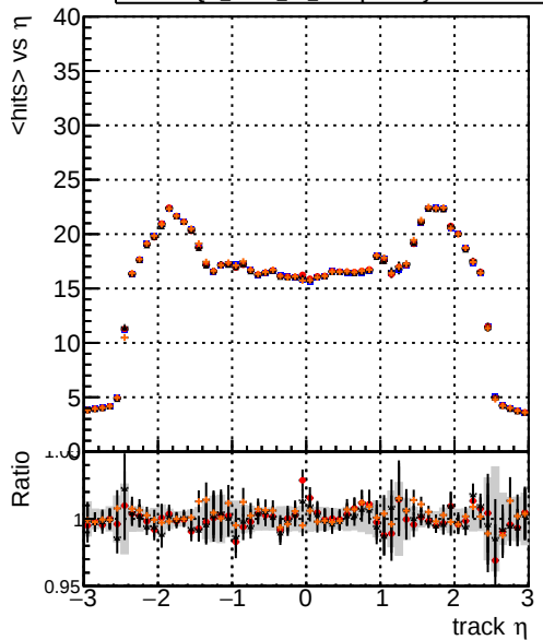
Legend: — DQM_mkFit_TT_original — DQM_mkFit_TT_JanUpdate-noErr — DQM_mkFit_TT_JanUpdate-statErr — DQM_mkFit_TT_JanUpdate-systErr mean hit
