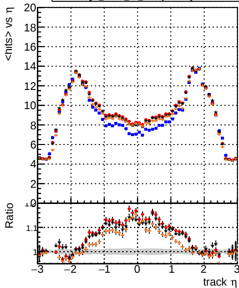
— DQM_mkFit_TT original — DQM_mkFit_TT_JanUpdate-noErr — DQM_mkFit_TT_JanUpdate-statErr — DQM_mkFit_TT_JanUpdate-systErr mean hit
