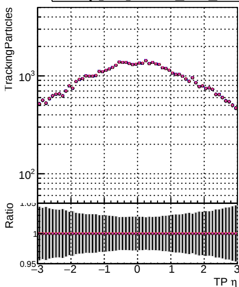
N of sin DQM V0001 R000 DQM V0001 R000 DQM V0001 R000
