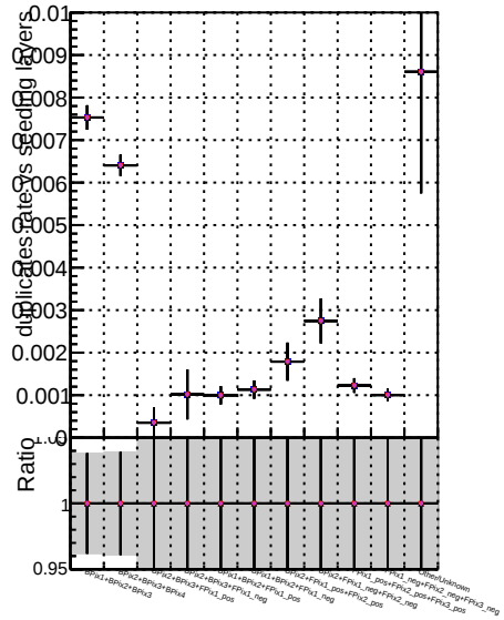
mkFit1000o RECO mkFit1000o ATime RECO mkFit1000o MTime RECO
