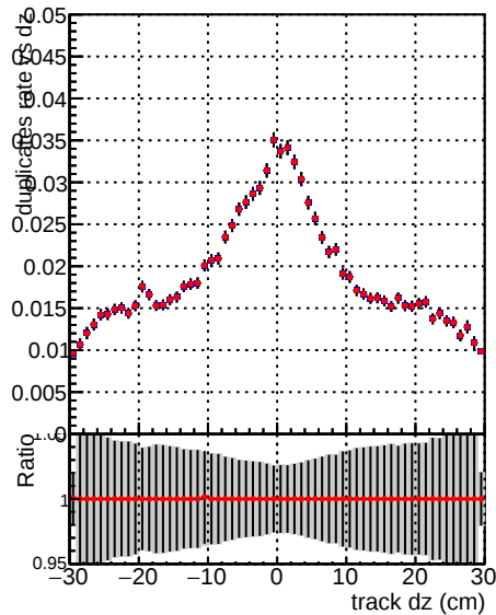
Global mkFit1000o RECO
