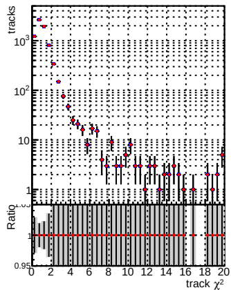
N of reco track vs. \chi^2 — Global mkFit1000o RECO — Global mkFit1000 RECO
