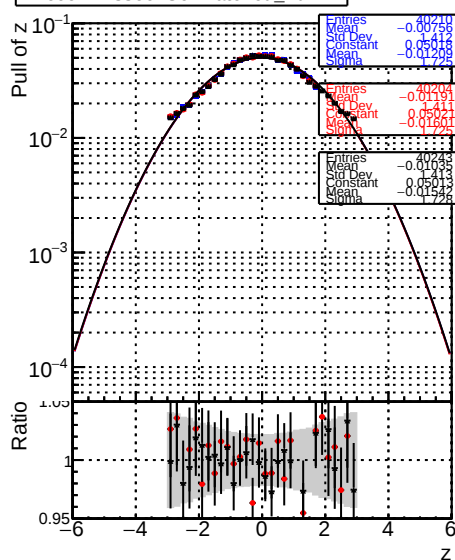
RecoAllAssoc2GenMatched_PullIZ
