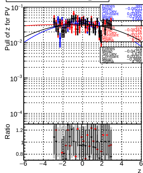
RecoPVAssoc2GenPVMatched_PullIZ
