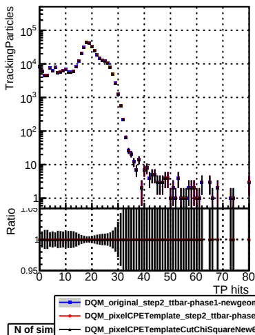
N of sim → DQM_pixelCPETemplateC
