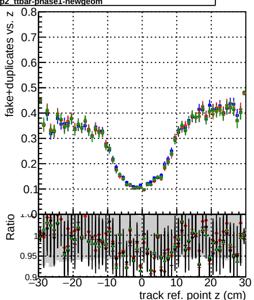
2 ttbar-phase1-newgeom 3 ttbar-phase1-newgeom 4 ttbar-phase1-newgeom
