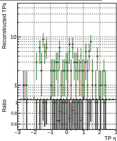
2 ttpar-phase1-newgeom 2 ttpar-phase1-newgeom 7 ttpar-phase1-newgeom
