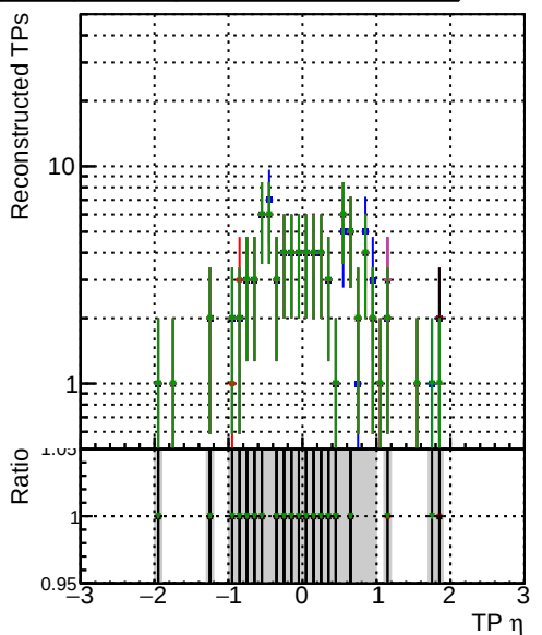
2 ttpar-phase1-newgeom 2 ttpar-phase1-newgeom 7 ttpar-phase1-newgeom
