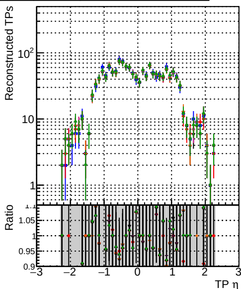
2- ttpar-phase1-newgeom 2- ttpar-phase1-newgeom
