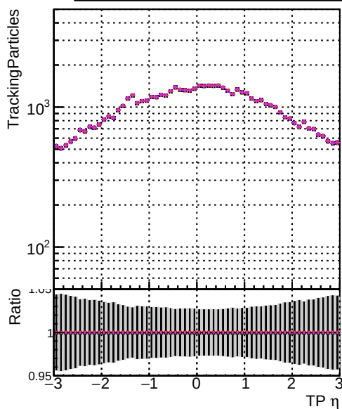
N of sim DOM pixel CP PET DOM pixel CP PET DOM pixel CP PET
