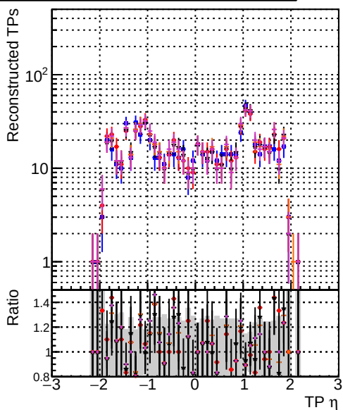
ttbar-phase1-newgeom 2 ttbar-phase1-newgeom 2 ttbar-phase1-newgeom
