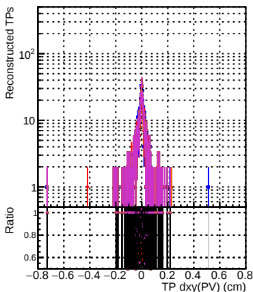
2 ttbar-phase1-newgeom 2 ttbar-phase1-newgeom
