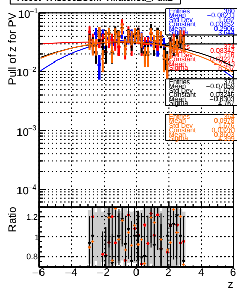
RecoPVAssoc2GenPVMatched_PullIZ
