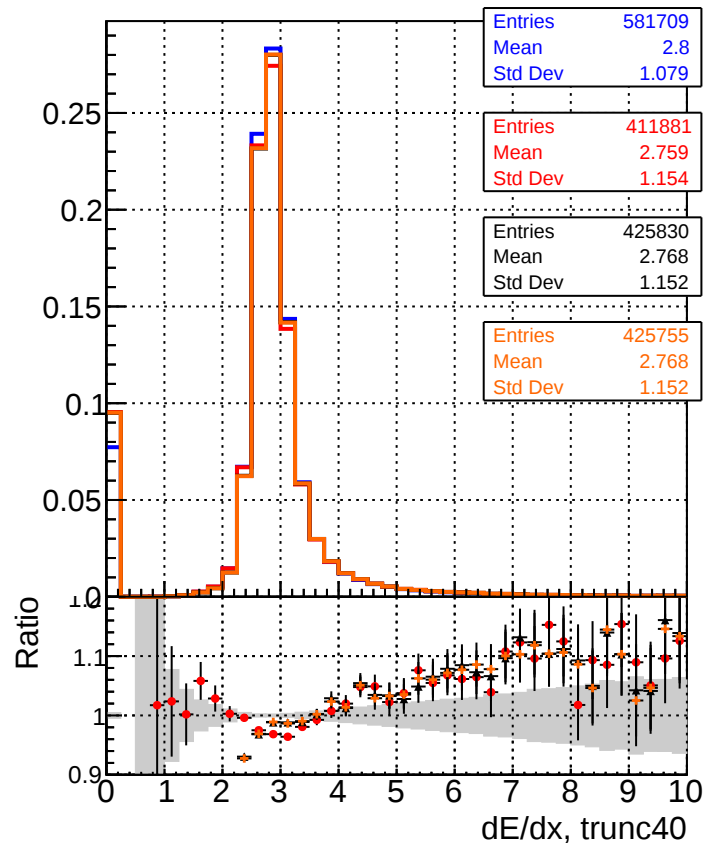
dE/dx estimator 2
