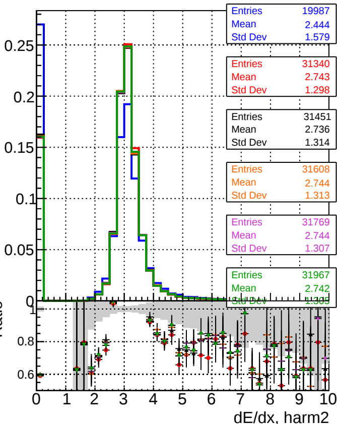
dE/dx estimator 1
