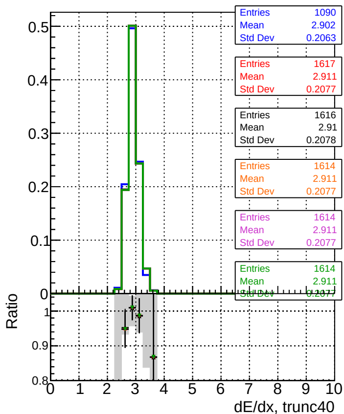
dE/dx estimator 2
