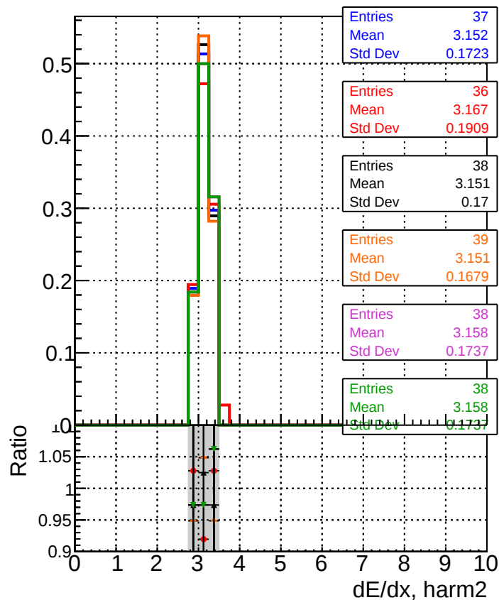
dE/dx estimator 1
