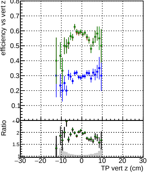
Efficiency vs vert z Legend: Blue line: B0 to eta1 eta2 eta3 eta4 eta5 eta6 eta7 eta8 eta9 eta10 eta11 eta12 eta13 eta14 eta15 eta16 eta17 eta18 eta19 eta20 eta21 eta22 eta23 eta24 eta25 eta26 eta27 eta28 eta29 eta30 eta31 eta32 eta33 eta34 eta35 eta36 eta37 eta38 eta39 eta40 eta41 eta42 eta43 eta44 eta45 eta46 eta47 eta48 eta49 eta50 eta51 eta52 eta53 eta54 eta55 eta56 eta57 eta58 eta59 eta60 eta61 eta62 eta63 eta64 eta65 eta66 eta67 eta68 eta69 eta70 eta71 eta72 eta73 eta74 eta75 eta76 eta77 eta78 eta79 eta80 eta81 eta82 eta83 eta84 eta85 eta86 eta87 eta88 eta89 eta90 eta91 eta92 eta93 eta94 eta95 eta96 eta97 eta98 eta99 eta100 eta101 eta102 eta103 eta104 eta105 eta106 eta107 eta108 eta109 eta110 eta111 eta112 eta113 eta114 eta115 eta116 eta117 eta118 eta119 eta120 eta121 eta122 eta123 eta124 eta125 eta126 eta127 eta128 eta129 eta130 eta131 eta132 eta133 eta134 eta135 eta136 eta137 eta138 eta139 eta140 eta141 eta142 eta143 eta144 eta145 eta146 eta147 eta148 eta149 eta150 eta151 eta152 eta153 eta154 eta155 eta156 eta157 eta158 eta159 eta160 eta161 eta162 eta163 eta164 eta165 eta166 eta167 eta168 eta169 eta170 eta171 eta172 eta173 eta174 eta175 eta176 eta177 eta178 eta179 eta180 eta181 eta182 eta183 eta184 eta185 eta186 eta187 eta188 eta189 eta190 eta191 eta192 eta193 eta194 eta195 eta196 eta197 eta198 eta199 eta200 eta201 eta202 eta203 eta204 eta205 eta206 eta207 eta208 eta209 eta210 eta211 eta212 eta213 eta214 eta215 eta216 eta217 eta218 eta219 eta220 eta221 eta222 eta223 eta224 eta225 eta226 eta227 eta228 eta229 eta230 eta231 eta232 eta233 eta234 eta235 eta236 eta237 eta238 eta239 eta240 eta241 eta242 eta243 eta244 eta245 eta246 eta247 eta248 eta249 eta250 eta251 eta252 eta253 eta254 eta255 eta256 eta257 eta258 eta259 eta260 eta261 eta262 eta263 eta264 eta265 eta266 eta267 eta268 eta269 eta270 eta271 eta272 eta273 eta274 eta275 eta276 eta277 eta278 eta279 eta280 eta281 eta282 eta283 eta284 eta285 eta286 eta287 eta288 eta289 eta290 eta291 eta292 eta293 eta294 eta295 eta296 eta297 eta298 eta299 eta300 eta301 eta302 eta303 eta304 eta305 eta306 eta307 eta308 eta309 eta310 eta311 eta312 eta313 eta314 eta315 eta316 eta317 eta318 eta319 eta320 eta321 eta322 eta323 eta324 eta325 eta326 eta327 eta328 eta329 eta330 eta331 eta332 eta333 eta334 eta335 eta336 eta337 eta338 eta339 eta340 eta341 eta342 eta343 eta344 eta345 eta346 eta347 eta348 eta349 eta350 eta351 eta352 eta353 eta354 eta355 eta356 eta357 eta358 eta359 eta360 eta361 eta362 eta363 eta364 eta365 eta366 eta367 eta368 eta369 eta370 eta371 eta372 eta373 eta374 eta375 eta376 eta377 eta378 eta379 eta380 eta381 eta382 eta383 eta384 eta385 eta386 eta387 eta388 eta389 eta390 eta391 eta392 eta393 eta394 eta395 eta396 eta397 eta398 eta399 eta400 eta401 eta402 eta403 eta404 eta405 eta406 eta407 eta408 eta409 eta410 eta411 eta412 eta413 eta414 eta415 eta416 eta417 eta418 eta419 eta420 eta421 eta422 eta423 eta424 eta425 eta426 eta427 eta428 eta429 eta430 eta431 eta432 eta433 eta434 eta435 eta436 eta437 eta438 eta439 eta440 eta441 eta442 eta443 eta444 eta445 eta446 eta447 eta448 eta449 eta450 eta451 eta452 eta453 eta454 eta455 eta456 eta457 eta458 eta459 eta460 eta461 eta462 eta463 eta464 eta465 eta466 eta467 eta468 eta469 eta470 eta471 eta472 eta473 eta474 eta475 eta476 eta477 eta478 eta479 eta480 eta481 eta482 eta483 eta484 eta485 eta486 eta487 eta488 eta489 eta490 eta491 eta492 eta493 eta494 eta495 eta496 eta497 eta498 eta499 eta500 eta501 eta502 eta503 eta504 eta505 eta506 eta507 eta508 eta509 eta510 eta511 eta512 eta513 eta514 eta515 eta516 eta517 eta518 eta519 eta520 eta521 eta522 eta523 eta524 eta525 eta526 eta527 eta528 eta529 eta530 eta531 eta532 eta533 eta534 eta535 eta536 eta537 eta538 eta539 eta540 eta541 eta542 eta543 eta544 eta545 eta546 eta547 eta548 eta549 eta550 eta551 eta552 eta553 eta554 eta555 eta556 eta557 eta558 eta559 eta560 eta561 eta562 eta563 eta564 eta565 eta566 eta567 eta568 eta569 eta570 eta571 eta572 eta573 eta574 eta575 eta576 eta577 eta578 eta579 eta580 eta581 eta582 eta583 eta584 eta585 eta586 eta587 eta588 eta589 eta590 eta591 eta592 eta593 eta594 eta595 eta596 eta597 eta598 eta599 eta600 eta601 eta602 eta603 eta604 eta605 eta606 eta607 eta608 eta609 eta610 eta611 eta612 eta613 eta614 eta615 eta616 eta617 eta618 eta619 eta620 eta621 eta622 eta623 eta624 eta625 eta626 eta627 eta628 eta629 eta630 eta631 eta632 eta633 eta634 eta635 eta636 eta637 eta638 eta639 eta640 eta641 eta642 eta643 eta644 eta645 eta646 eta647 eta648 eta649 eta650 eta651 eta652 eta653 eta654 eta655 eta656 eta657 eta658 eta659 eta660 eta661 eta662 eta663 eta664 eta665 eta666 eta667 eta668 eta669 eta670 eta671 eta672 eta673 eta674 eta675 eta676 eta677 eta678 eta679 eta680 eta681 eta682 eta683 eta684 eta685 eta686 eta687 eta688 eta689 eta690 eta691 eta692 eta693 eta694 eta695 eta696 eta697 eta698 eta699 eta700 eta701 eta702 eta703 eta704 eta705 eta706 eta707 eta708 eta709 eta710 eta711 eta712 eta713 eta714 eta715 eta716 eta717 eta718 eta719 eta720 eta721 eta722 eta723 eta724 eta725 eta726 eta727 eta728 eta729 eta730 eta731 eta732 eta733 eta734 eta735 eta736 eta737 eta738 eta739 eta740 eta741 eta742 eta743 eta744 eta745 eta746 eta747 eta748 eta749 eta750 eta751 eta752 eta753 eta754 eta755 eta756 eta757 eta758 eta759 eta760 eta761 eta762 eta763 eta764 eta765 eta766 eta767 eta768 eta769 eta770 eta771 eta772 eta773 eta774 eta775 eta776 eta777 eta778 eta779 eta780 eta781 eta782 eta783 eta784 eta785 eta786 eta787 eta788 eta789 eta790 eta791 eta792 eta793 eta794 eta795 eta796 eta797 eta798 eta799 eta800 eta801 eta802 eta803 eta804 eta805 eta806 eta807 eta808 eta809 eta810 eta811 eta812 eta813 eta814 eta815 eta816 eta817 eta818 eta819 eta820 eta821 eta822 eta823 eta824 eta825 eta826 eta827 eta828 eta829 eta830 eta831 eta832 eta833 eta834 eta835 eta836 eta837 eta838 eta839 eta840 eta841 eta842 eta843 eta844 eta845 eta846 eta847 eta848 eta849 eta850 eta851 eta852 eta853 eta854 eta855 eta856 eta857 eta858 eta859 eta860 eta861 eta862 eta863 eta864 eta865 eta866 eta867 eta868 eta869 eta870 eta871 eta872 eta873 eta874 eta875 eta876 eta877 eta878 eta879 eta880 eta881 eta882 eta883 eta884 eta885 eta886 eta887 eta888 eta889 eta890 eta891 eta892 eta893 eta894 eta895 eta896 eta897 eta898 eta899 eta900 eta901 eta902 eta903 eta904 eta905 eta906 eta907 eta908 eta909 eta910 eta911 eta912 eta913 eta914 eta915 eta916 eta917 eta918 eta919 eta920 eta921 eta922 eta923 eta924 eta925 eta926 eta927 eta928 eta929 eta930 eta931 eta932 eta933 eta934 eta935 eta936 eta937 eta938 eta939 eta940 eta941 eta942 eta943 eta944 eta945 eta946 eta947 eta948 eta949 eta950 eta951 eta952 eta953 eta954 eta955 eta956 eta957 eta958 eta959 eta960 eta961 eta962 eta963 eta964 eta965 eta966 eta967 eta968 eta969 eta970 eta971 eta972 eta973 eta974 eta975 eta976 eta977 eta978 eta979 eta980 eta981 eta982 eta983 eta984 eta985 eta986 eta987 eta988 eta989 eta990 eta991 eta992 eta993 eta994 eta995 eta996 eta997 eta998 eta999
