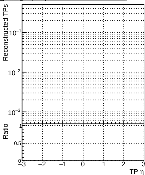
pt1to20 eta1p4to1p6 pt1to20 eta1p4to1p6 pt1to20 eta1p4to1p6 pt1to20 eta1p4to1p6
