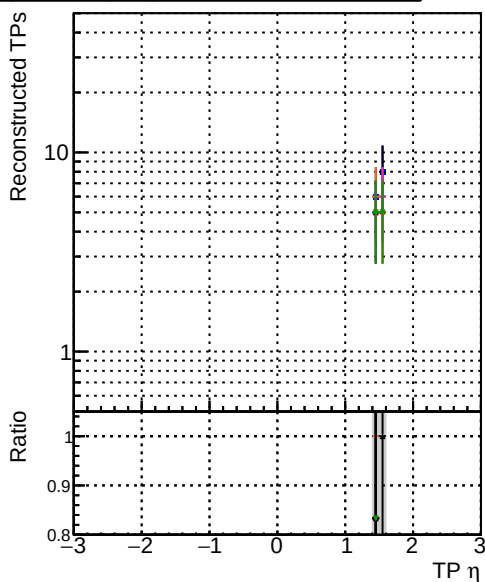
pt1to20-eta1p4to1p66 pt1to20-eta1p4to1p66 pt1to20-eta1p4to1p66
