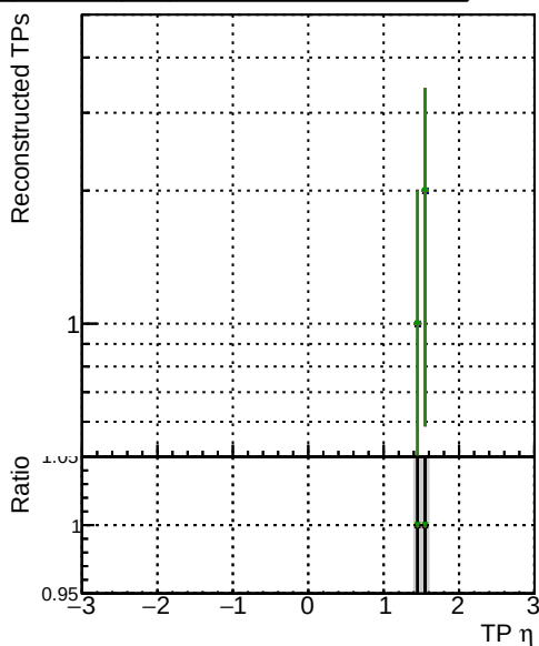
pt1to20-eta1p4to1p6
