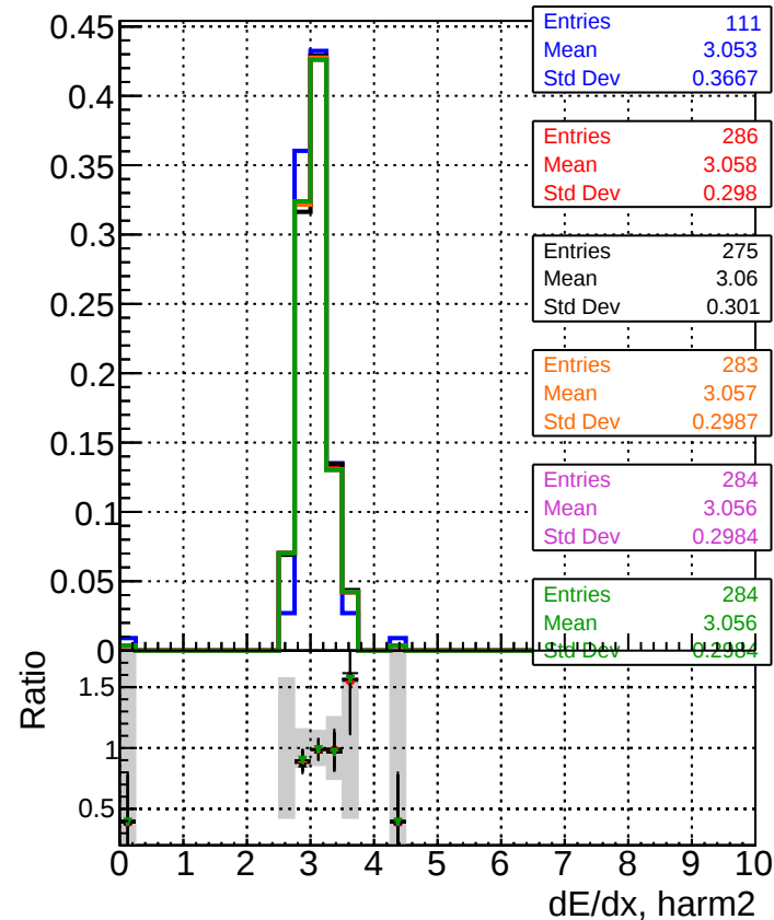
dE/dx estimator 1
