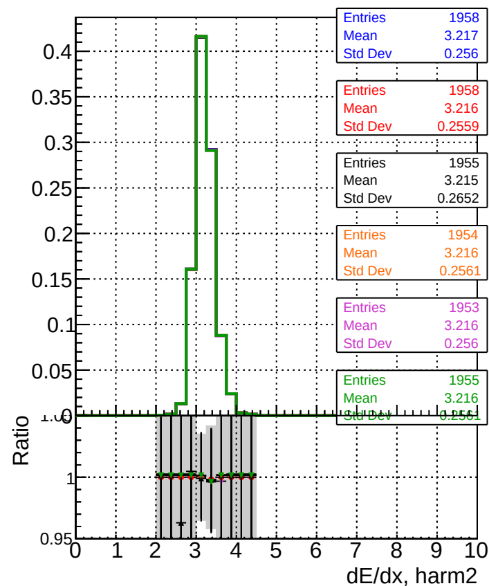
dE/dx estimator 1
