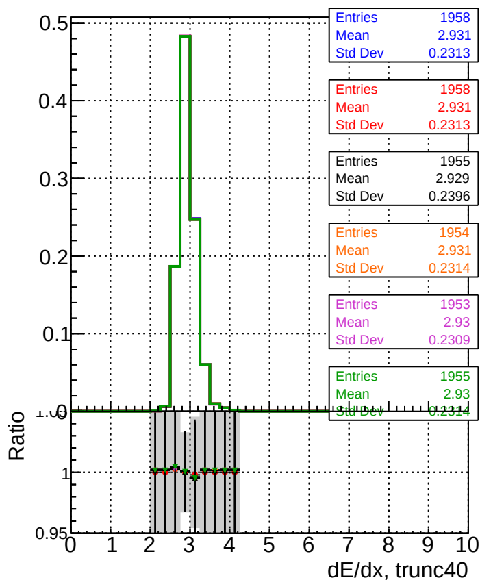
dE/dx estimator 2
