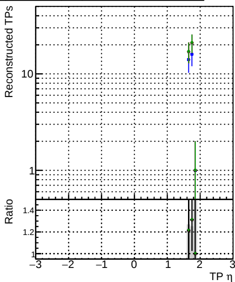
pt1to1000-eta1b6to2b0 pt1to1000-eta1b6to2b0
