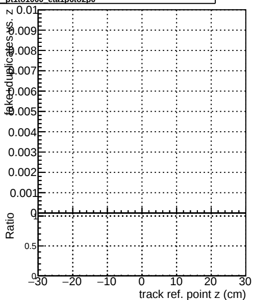
pt1to1000-eta1b6to2b0 pt1to1000-eta1b6to2b0 pt1to1000-eta1b6to2b0 pt1to1000-eta1b6to2b0
