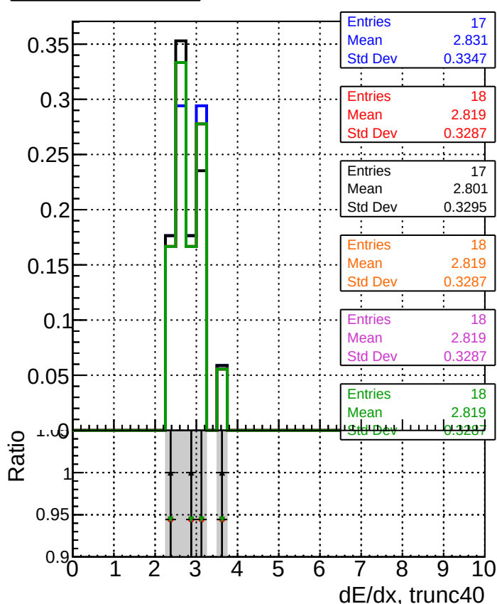
dE/dx estimator 2
