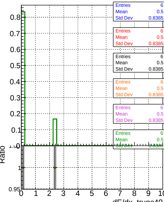
dE/dx estimator 2
