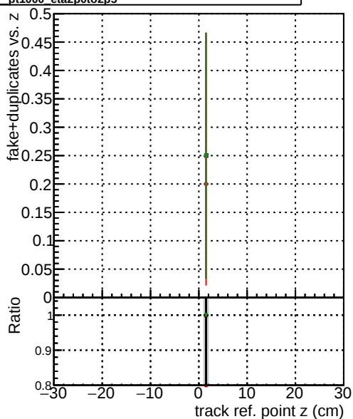
pt1000 eta2 b0t02 b5 pt1000 eta2 b0t02 b5 pt1000 eta2 b0t02 b5
