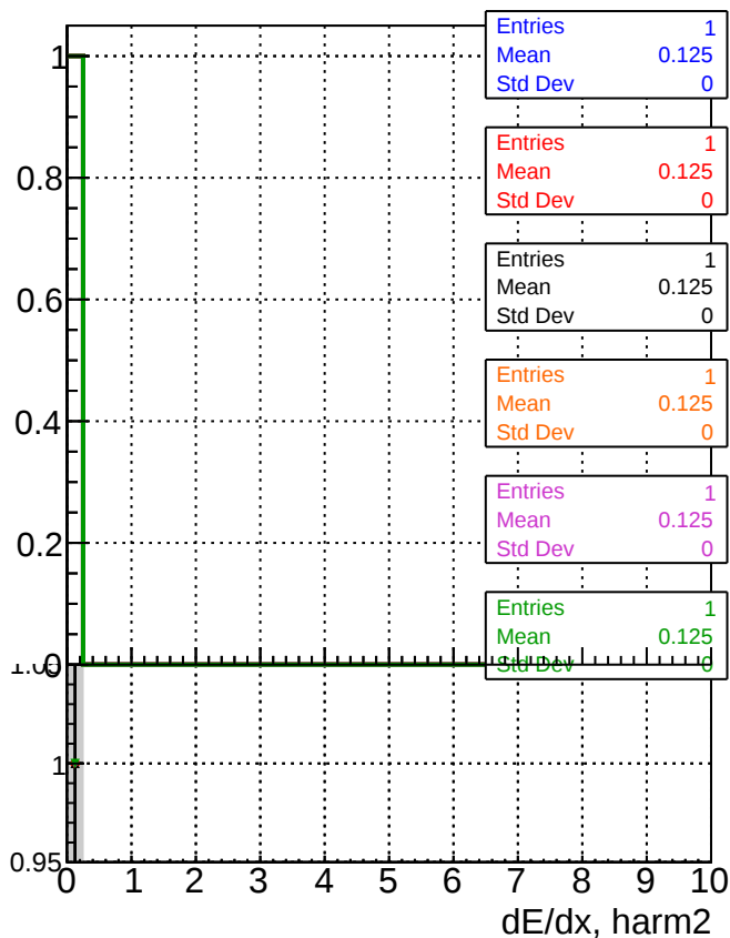
dE/dx estimator 1
