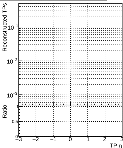
pt0p1t01-eta2p0t02p5p5 pt0p1t01-eta2p0t02p5p5
